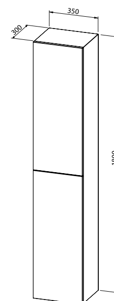
Hochschrank 35x180 , 2 Türen, universal - Öffnen durch Berührung - 5 Regale
