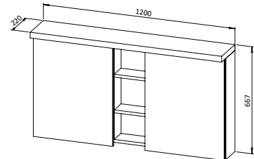
Hängeschränkchen ASTRA 120 mit Spiegel und LED-Beleuchtung, 2 Türen, Einlegeböden - 2 Regale - Schalter und Steckdose (Powerbox)
