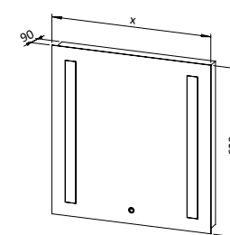
Spiegel mit integrierter Beleuchtung, 2 Streifen 45, 60, 80, 100, 120 - Steckdose, Touch-Schalter, LED-Beleuchtung, Antibeschlagheizung
