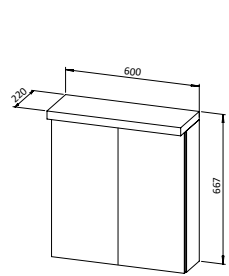
Hängeschränkchen ASTRA 60 mit Spiegel und LED Beleuchtung, 2 Türen - 1 Regal - Schalter und Steckdose (Powerbox)
