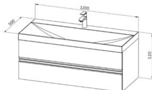
LYRA 120, 2 Schubladen OPTION: 2 Hahnlöcher
