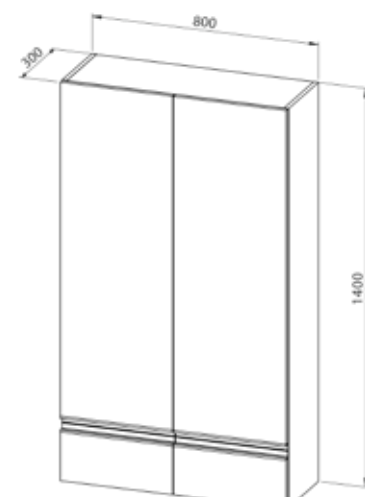
Hochschrank LYRA 80x140, 2 Türen, 2 Schubladen, universell - 4 Regale (x2)
