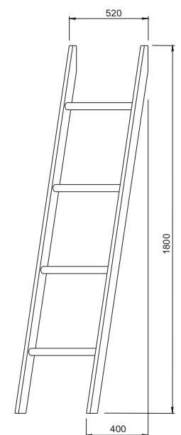
Handtuchleiter aus Holz 52x180 cm - weiß / schwarze Farbe - Montage an der Wand
