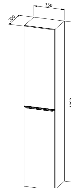
Hochschrank GRANDE 35x180 , 2 Türen, universal - 5 Regale
