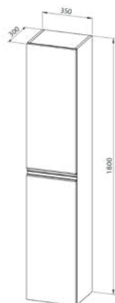
Hochschrank LYRA 35x180, 2 Türen, L/R - 4 Regale
