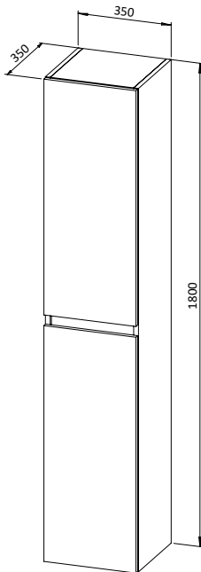
Hochschrank STELLA 35x180, 2 Türen, universal - 3 Regale
