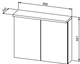
Hängeschränkchen ASTRA 80 mit Spiegel und LED Beleuchtung, 2 Türen - 2 Regale - Schalter und Steckdose (Powerbox)
