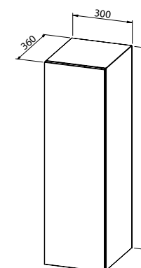
Halbhochschrank 30x100 , 1 Tür, universal - Öffnen durch Berührung - 2 Regale
