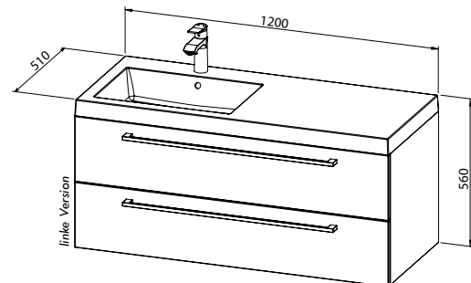
ARWEN 120, 2 Schubladen, L/R
