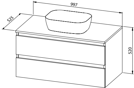
STELLA TOP 100 , 2 Schubladen OPTION: ohne Hahnloch
