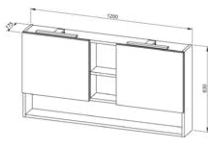
Hängeschränk BASIC PLUS 120 - LED-Beleuchtung - Schalter und Steckdose im Schrank - 2 Innenregale und 1 Außenregal
