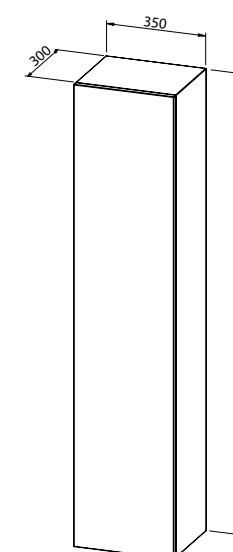
Hochschrank 35x160 , 1 Tür, universal - Öffnen durch Berührung - 4 Regale
