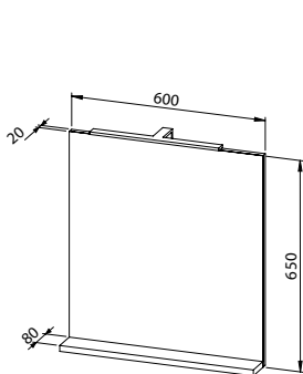
Spiegel STELLA 40, 50, 60, 70, 80, 90, 100 mit Lampe, Ablage und Schalter
