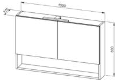
Hängeschränk BASIC PLUS 100 - LED-Beleuchtung - Schalter und Steckdose im Schrank - 2 Regale
