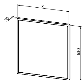
Spiegel mit Al-Rahmen 40, 60, 80, 90, 100, 120 - Rahmen silber/schwarz matt
